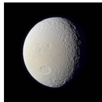
Gibbous moon
